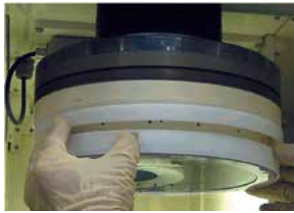
スナップリングを親指で広げる リテーナは落ちる
