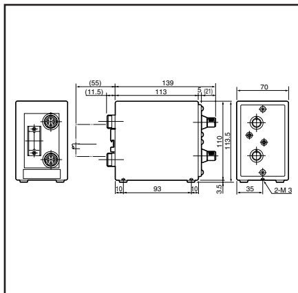
■ 外観寸法図
